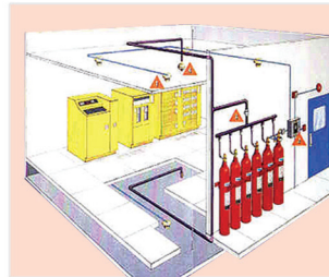
Fire extinguishing system نظام إطفاء الحريق
